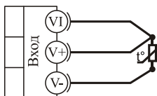
термометр сопротивления
