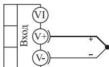
термопара
